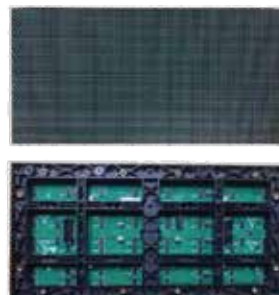
屋外用 LED モジュール
