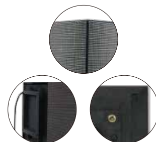
屋内用 P2.5 モジュール
